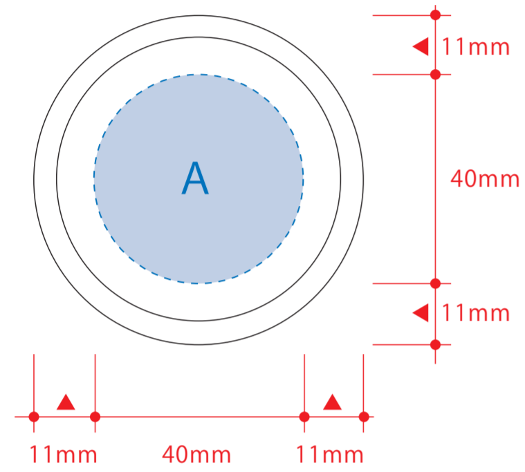
天面 (蓋)
